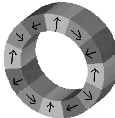
Halbach array
